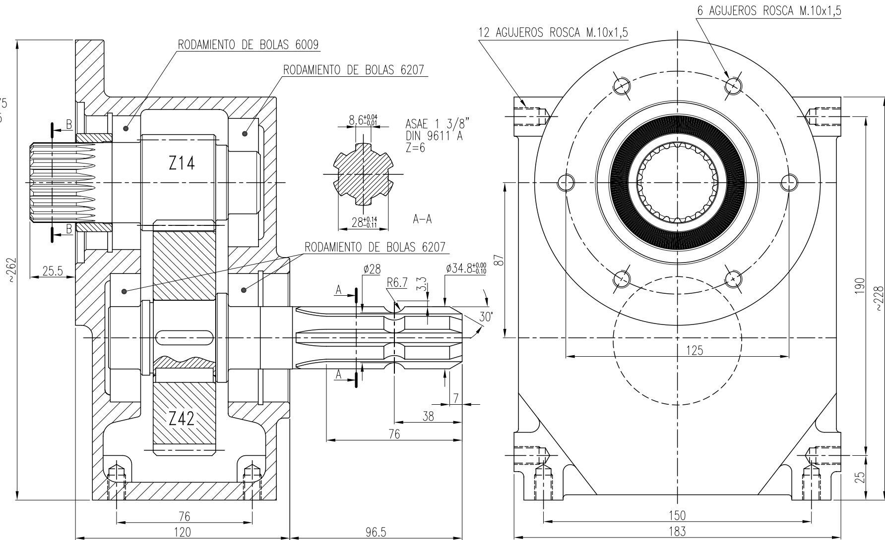
Corte B-B
