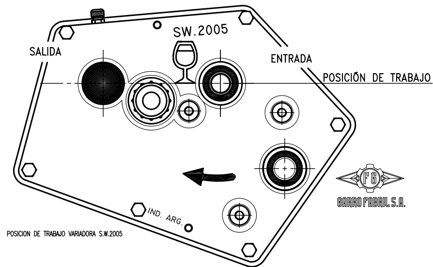
VISTA DE LA POSICION DE LA CAJA EN LA MAQUINA
